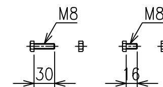
骨線取付金具 S=1/2
