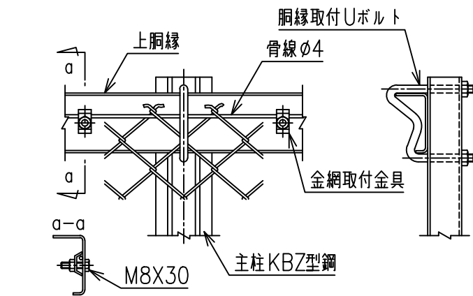
主柱胴縁取付部 S=1/6
