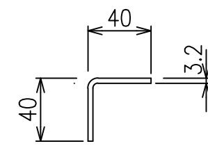
下胴縁 S=1/3
