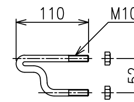
胴縁取付Uボルト S=1/5
