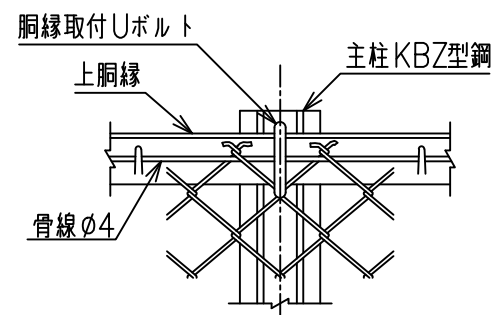
主柱胴縁取付部 S=1/6
