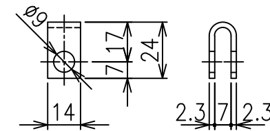
骨線取付金具 S=1/2
