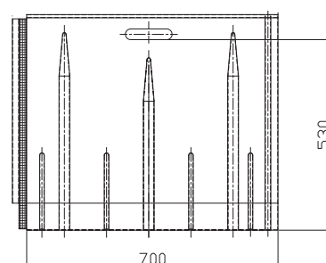
【正面図】
