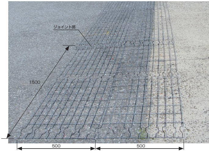
1.メッシュパネル (1500×500) を地面に2列配置 (パネル半円加工部 (ジョイント部) が重なるよう配置)
